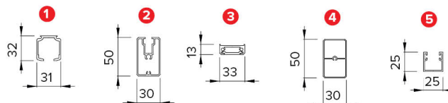
1 Binario superiore. 2 Profilo portante. 3 Telaio laterale doghe. 4 Profilo doga alluminio. 5 Binario inferiore. 1 Top rail. 2 Main profile. 3 Slats side frame. 4 Aluminium slat profile. 5 Bottom rail.
